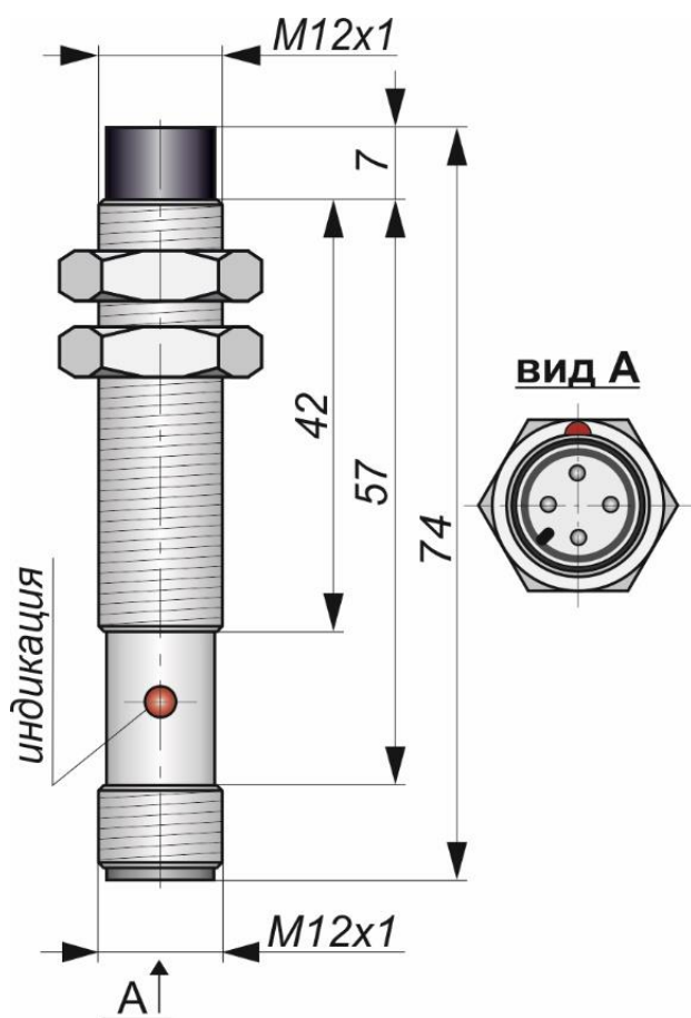
Габаритный чертеж
